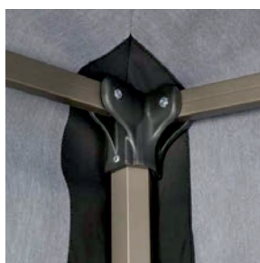
Robuste und stabile Eckgelenke
